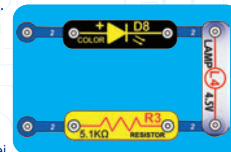
Przykład obwodu połączony szeregowo
